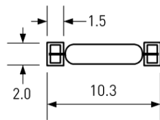
Löt pads
